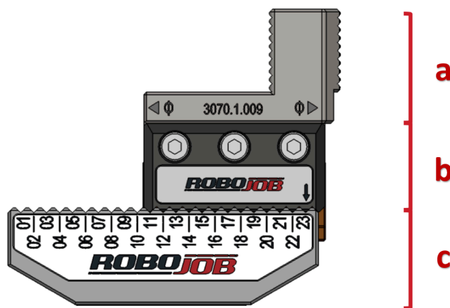
Abbildung 3.80. Teile der Greiferbacke
