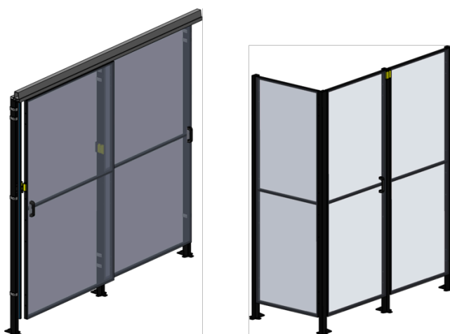
Abbildung 2.14. Sicherheits-Absperrung mit Schiebetüren (links) oder mit einer Klapptür (rechts)
