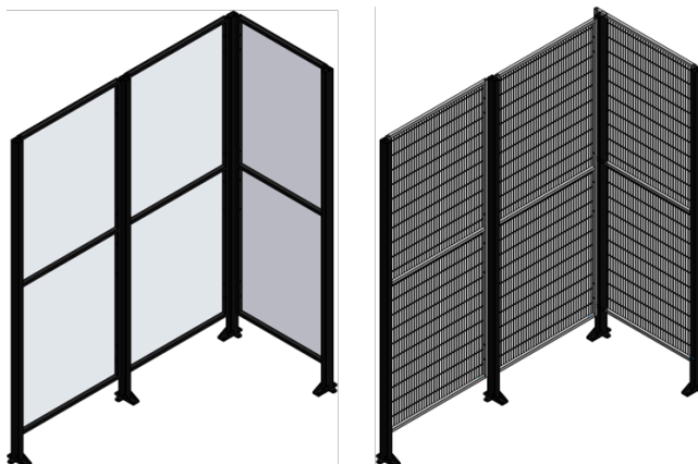
Abbildung 2.13. Sicherheits-Absperrung mit durchsichtigen Polycarbonat-Platten (links) oder mit Gitterplatten (rechts)
