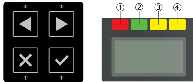
Abbildung 2.11. Anzeige- und Bedienelemente beim microScan3: Knöpfe (links) und Display (rechts)
