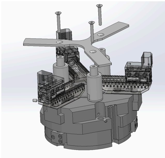
Abbildung 2.10. Teileschieber
