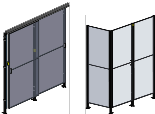
Abbildung 2.17. Sicherheits-Absperrung mit Schiebetüren (links) oder mit einer Klapptür (rechts)
