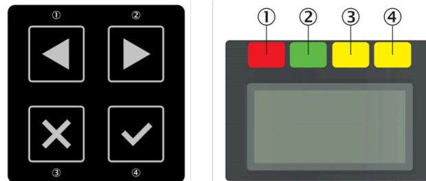
Abbildung 2.14. Anzeig- und Bedienelemente beim microScan3: Knöpfe (links) und Display (rechts)
