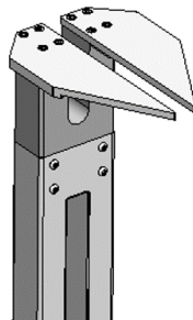
Abbildung 2.6. Wendeeinheit für Werkstücken auf einem Turn-Assist
